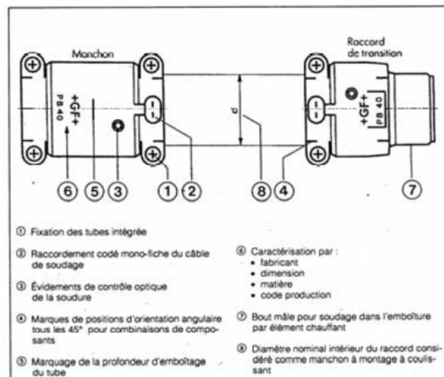
Figure 5 - Raccords électrosoudables
