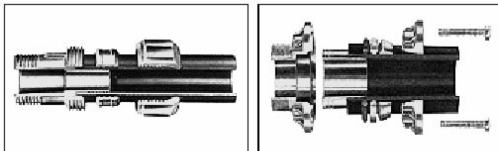
Figure 5 : Raccords à compression Beulco
